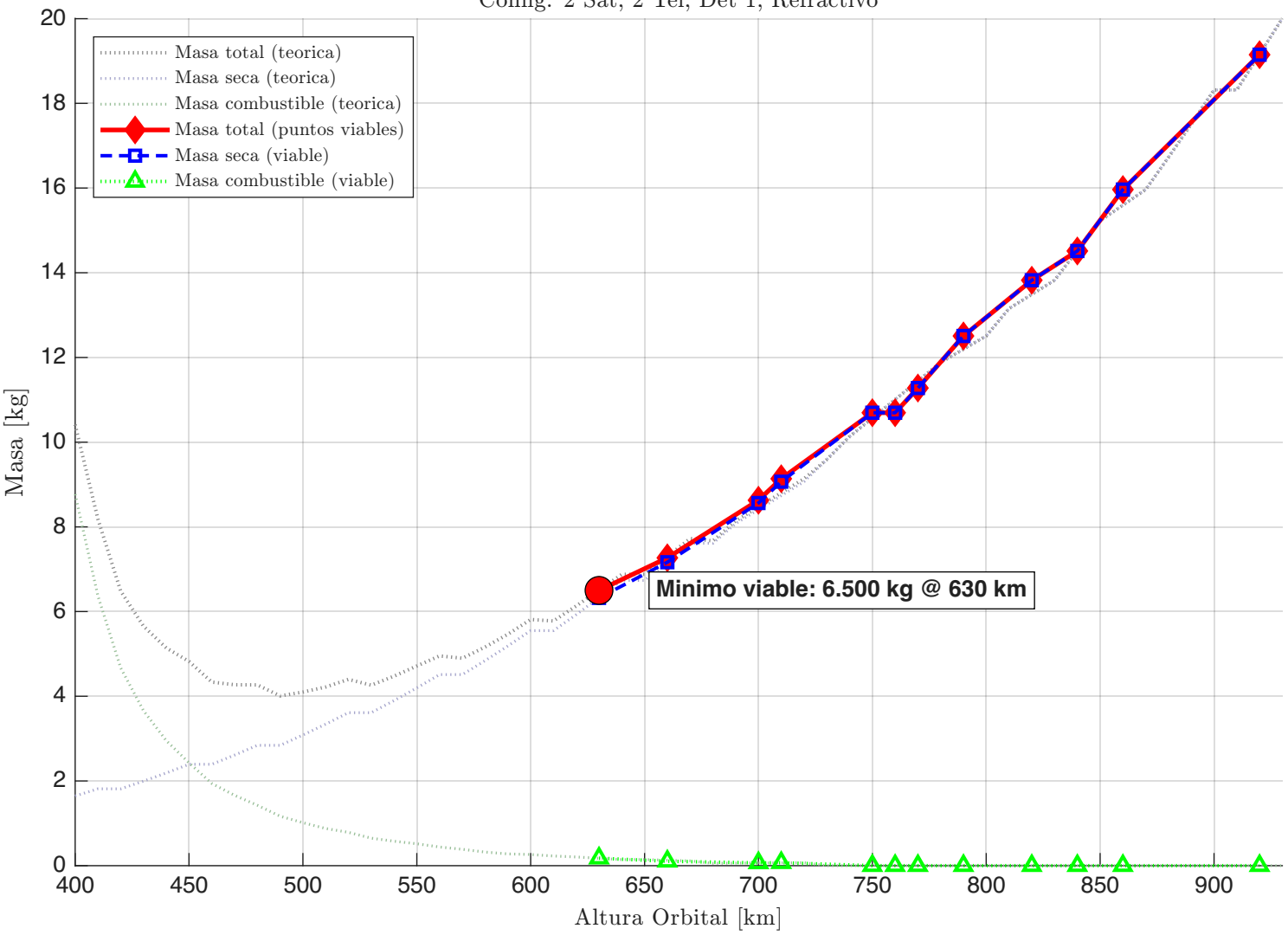
Desglose de Masas vs. Altura Config: 2 Sat, 2 Tel, Det 1, Refractivo
